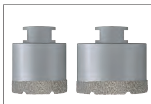
1x DBV 50x35 M14 15x3 1x DBV 65x35 M14 15x3
